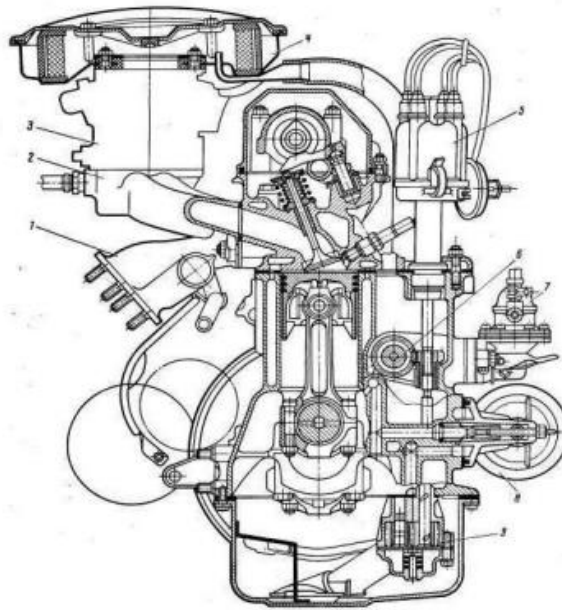
Рисунок 1 – Двигатель внутреннего сгорания в разрезе
