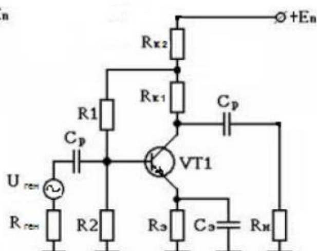
схема 2
