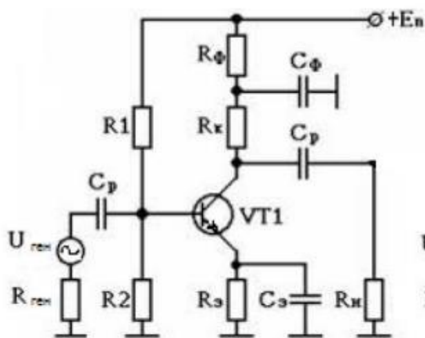
схема 1
