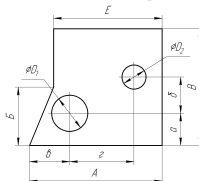
Рисунок 1 — Эскиз детали к заданию 2.1.1
