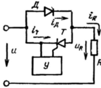
Рисунок 11 – Однофазный прерыватель переменного тока со схемой соединений «тиристор – диод»
