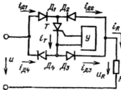
Рисунок 12 – Однофазный мостовой прерыватель переменного тока
