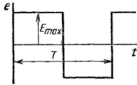
Рисунок 2 – Периодическое напряжение
