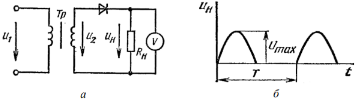
Рисунок 3 – Однополупериодный выпрямитель
