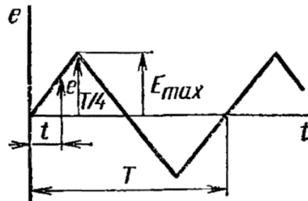
Рисунок 1 – Периодическая ЭДС
