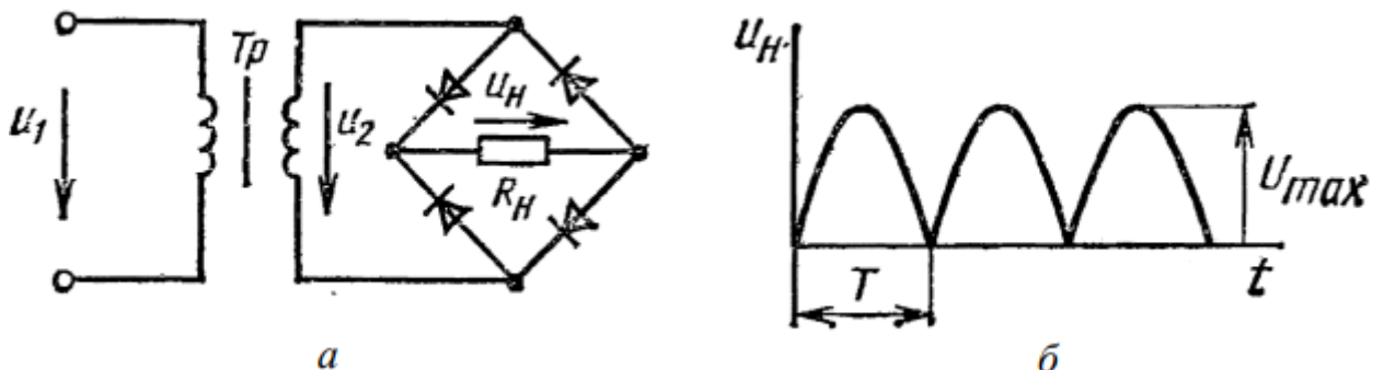
Рисунок 4 – Двухполупериодный выпрямитель
