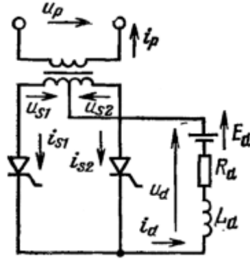
Рисунок 7 – Управляемый преобразователь со схемой 1Ф1Н2П
