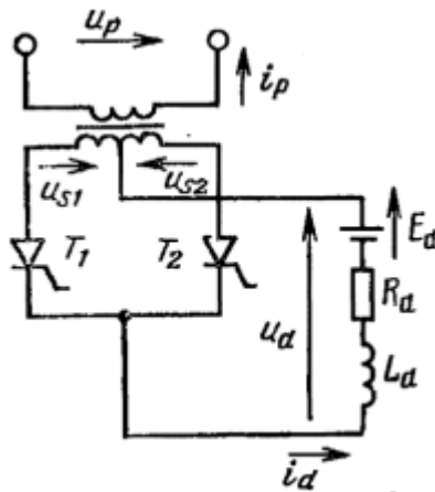
Рисунок 8 – Управляемый преобразователь со схемой 1Ф1Н2П
