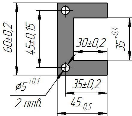
Материал: АМг5М ГОСТ 3836-73 s=2,5
