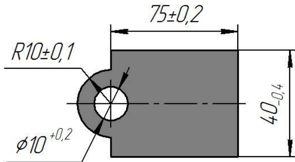
Материал: Сталь 30XGSA ГОСТ 4543-71 s=3
