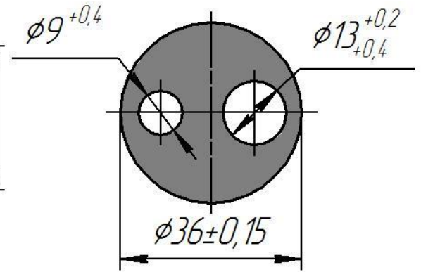
Материал: Сталь 20 ГОСТ 1050-88 s=2
