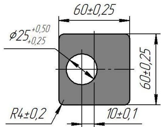
Материал: Сталь 10kp ГОСТ 1050-88 s=2
