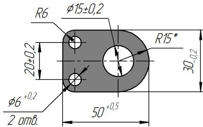
Материал: Сталь 15kp ГОСТ 1050-88 s=3
